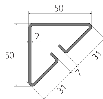
SEZIONE GAMBA
